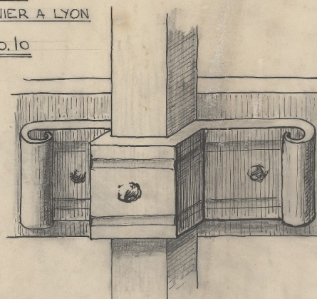
DETAIL FIXATION BARREAUX SUR TRAVERSES
